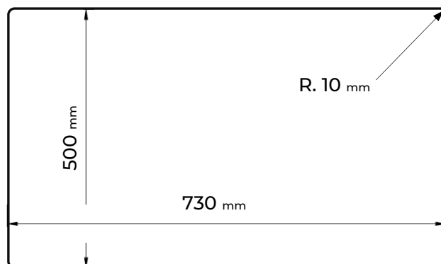
Sagoma di taglio del piano lavoro
