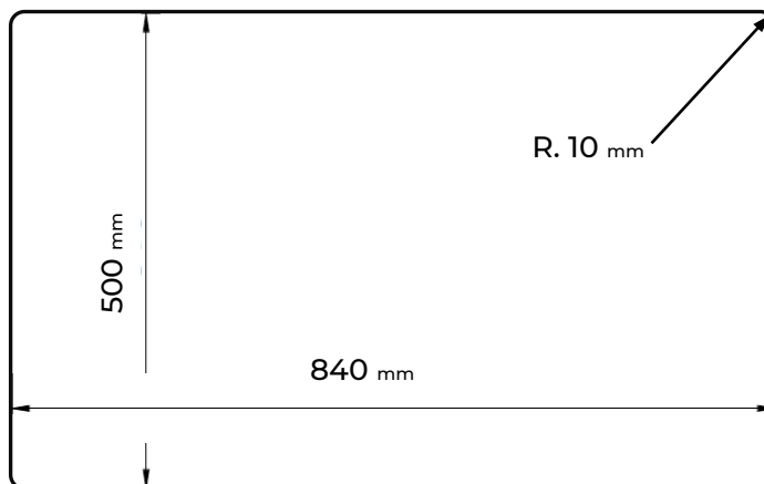
Sagoma di taglio del piano lavoro
