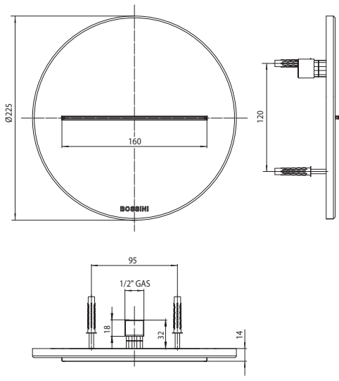
E89610 - Ø225 MM
