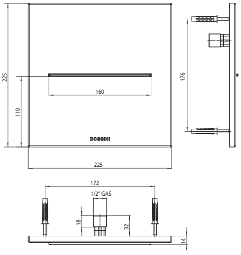
E89612 - 225x225 MM
